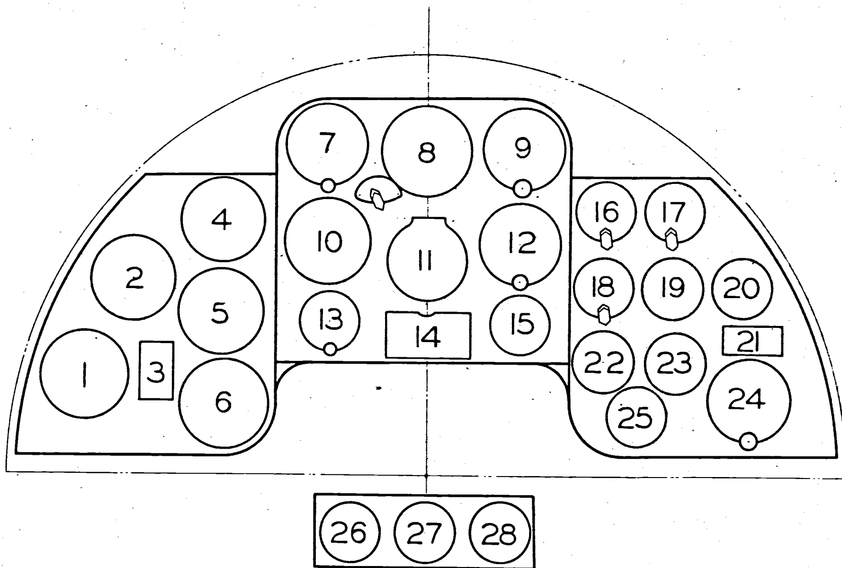
FIG. 29. INSTRUMENT LAYOUT.
